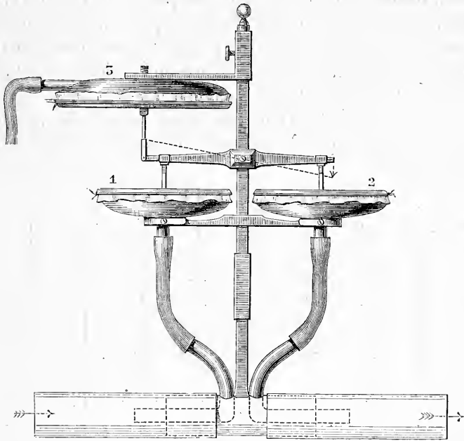
Fig. 144. — Appareil destiné à mesurer la vitesse du liquide dans un tube ou dans une artère.
